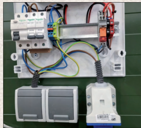
230V STROMANSCHLUSS ZUM BETRIEB EXTERNER GERÄTE
